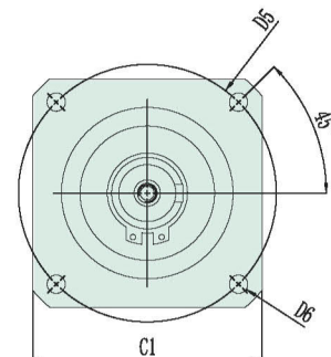
輸出端 Output
